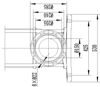
法兰PN16/DN150
