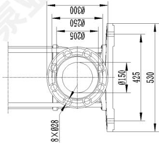
法兰PN25-40/DN150
